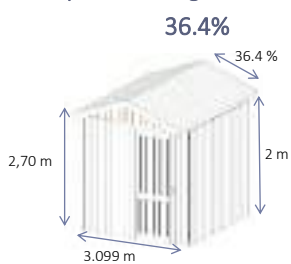
2 pentes shingle et bac acier
