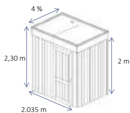
Toit plat Epdm 4%
