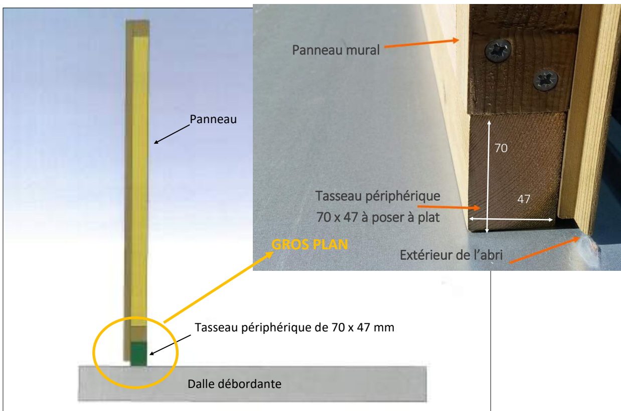
Pose sur dalle débordante
