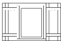
Châssis à la française AVEC ou SANS volets 59 cm x 77 cm
